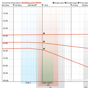
YSHIELD® HSF64
